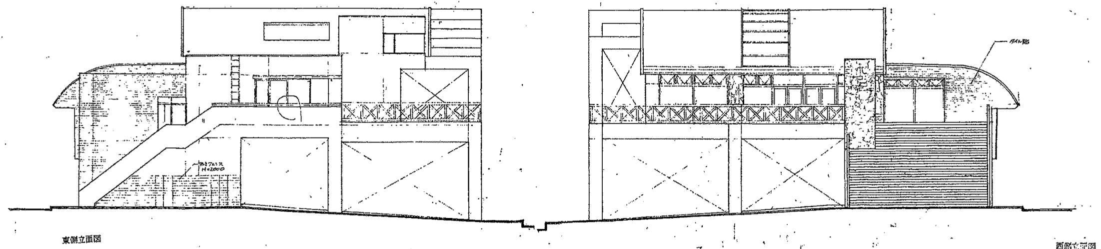
西側立面図
