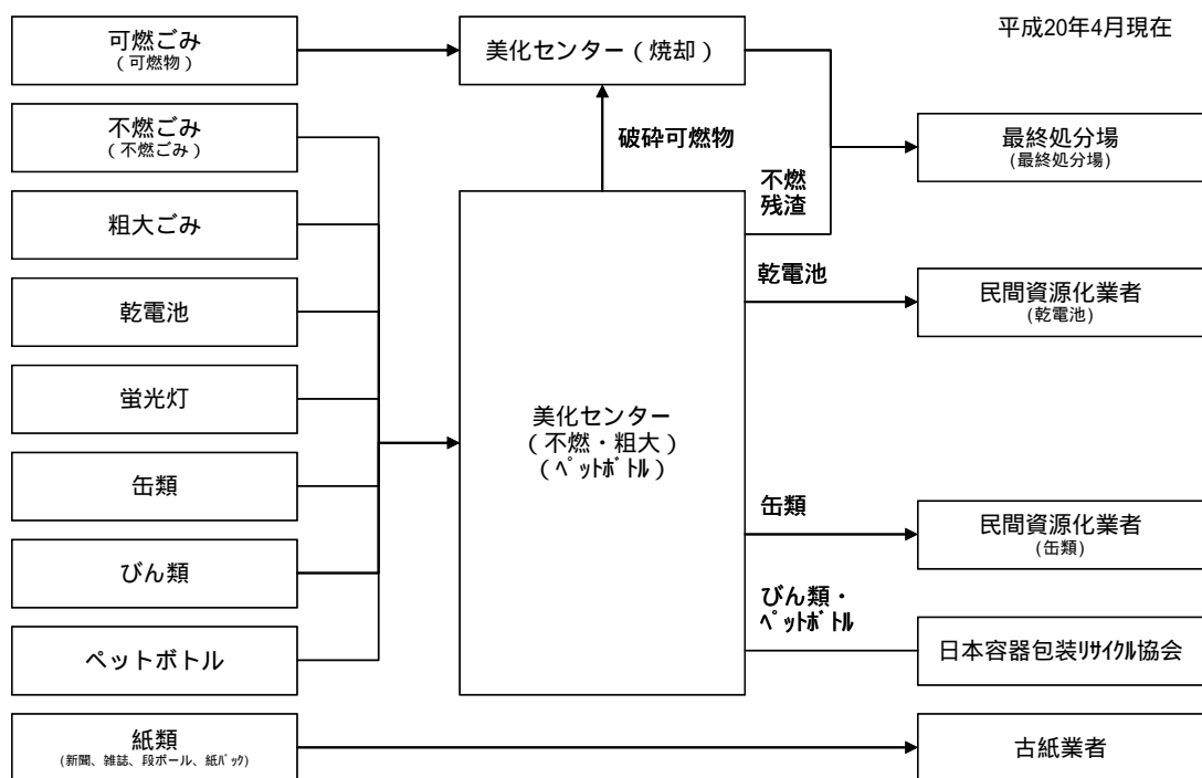
図5 湯河原町・真鶴町衛生組合のごみ処理フロー
